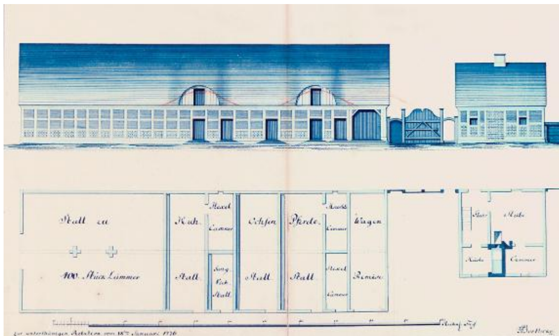
Lakoma (→ 3094), Umbau der Wirtschaftsgebäude auf dem Vorwerk, kol. Zeichnung von Boethcke, 1776
