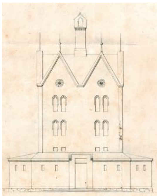
Seese (-> 4950), Fassade und Grundriss des Federviehstalles, 1861
