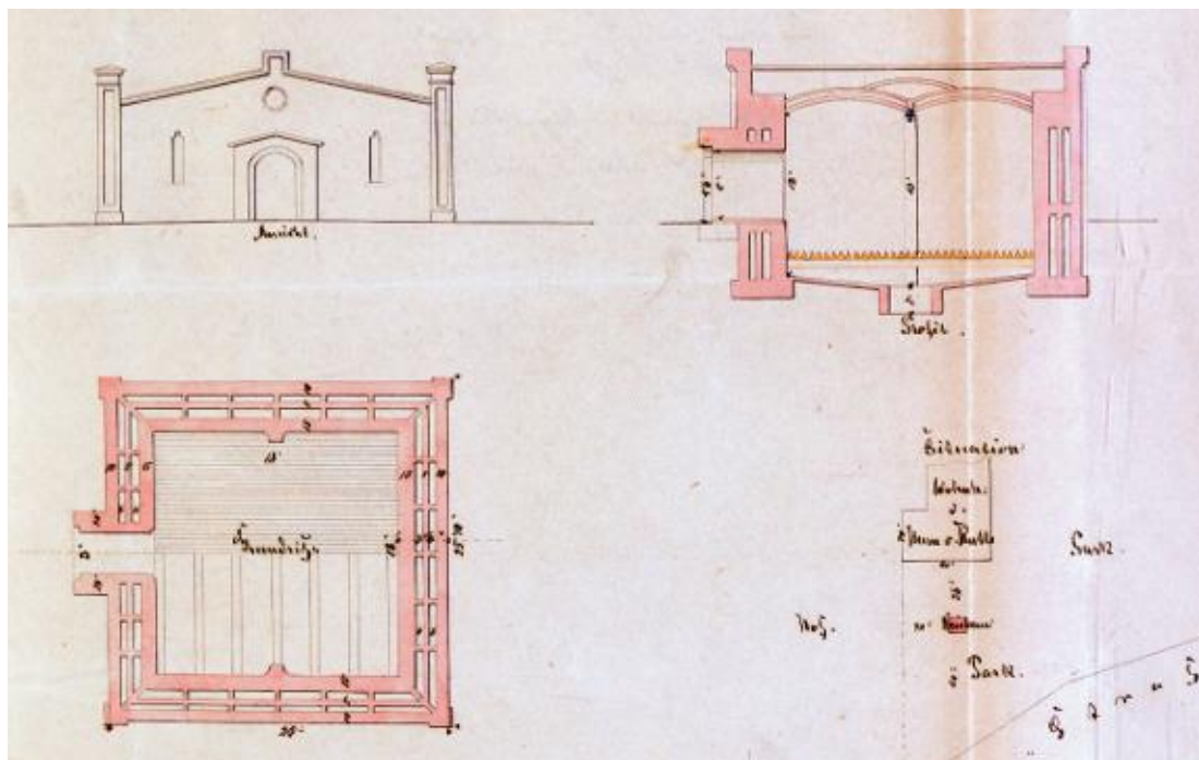
Roskow (→ 4596), Bauzeichnungen für einen Eiskeller (Ausschnitt), 1868
