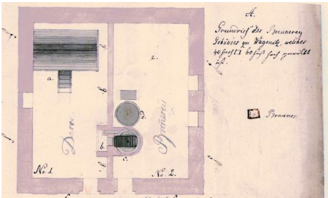
Wagenitz (→ 5499), Grundriß und Profil der Brennerei, 1814
