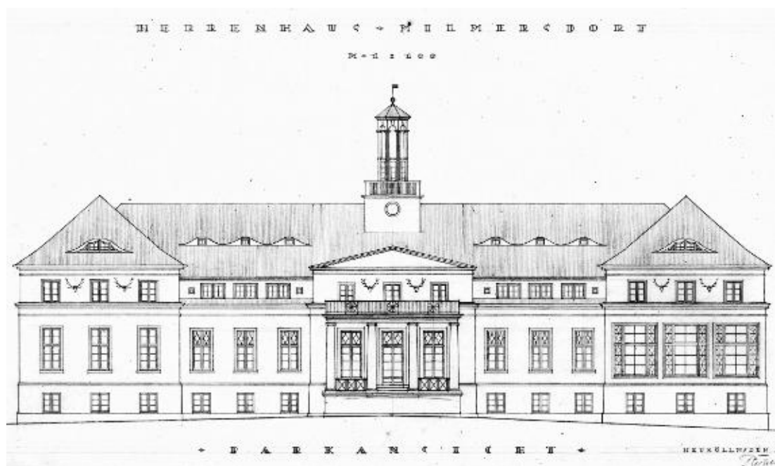
Milnersdorf (→ 3710), Umbau des Herrenhauses, Entwurf von C. Reichelt, 1919
