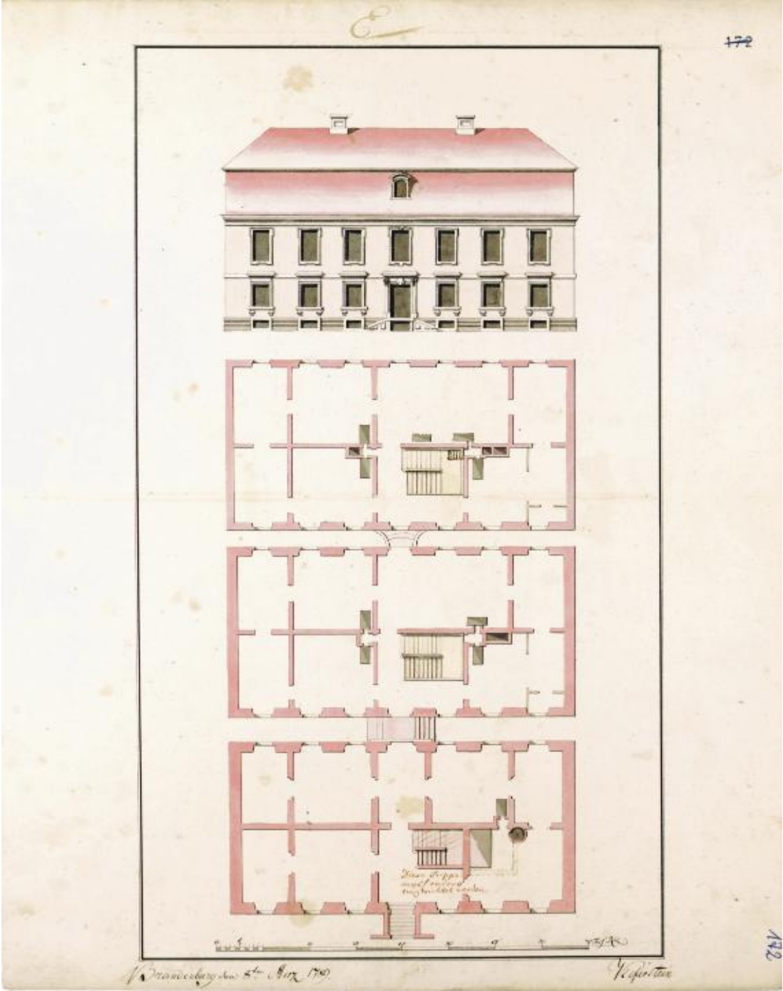
Priort (→ 4461), Grund- und Aufriss des Herrenhauses, kol. Zeichnung von Kefenstein, 1789
