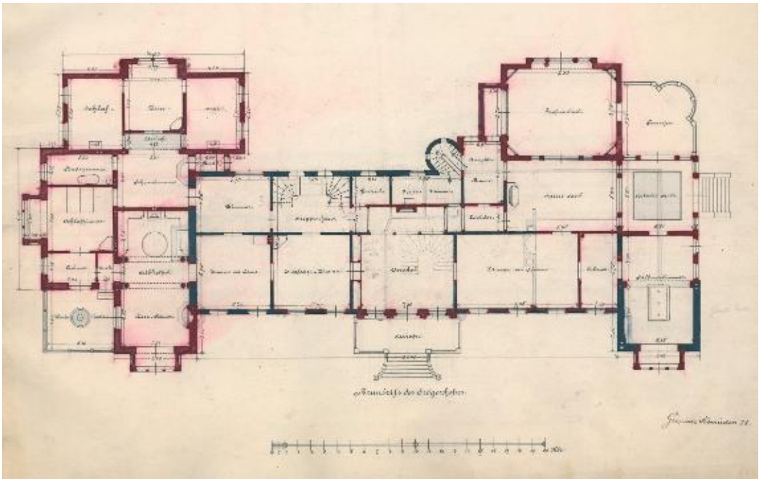
Karnzow (→ 2615), Umbau des Schlosses, Zeichnung von Gropius u. Schmieden, Berlin, 1878
